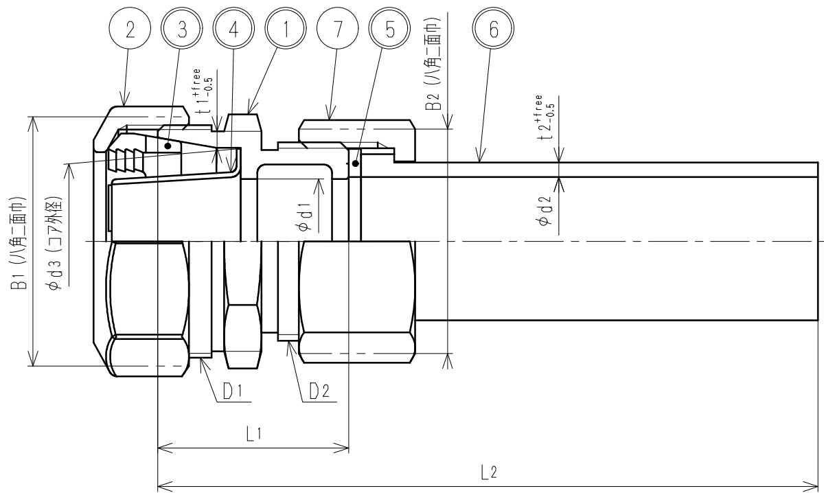
寸法表
